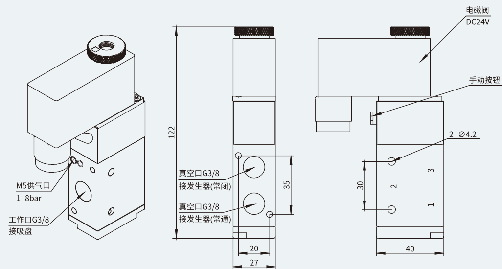
气路连接图
