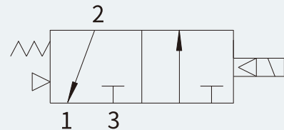
气路连接图
